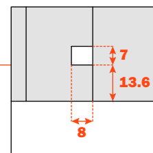
Lavorazione per il fissaggio della guida sul fianco del mobile
