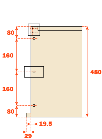
Lavorazione per il fissaggio del sistema sul fianco del mobile
