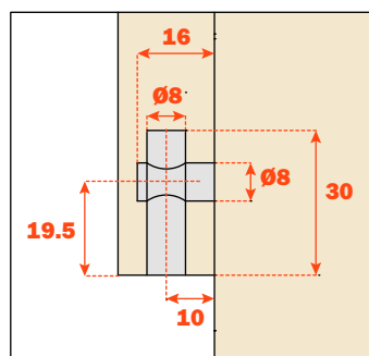
Lavorazione per il fissaggio della guida sul fianco da 19/20 mm
