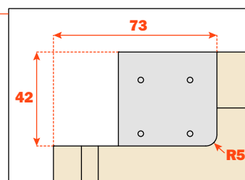
Lavorazione per l'incasso del sistema sulle spalle interne
