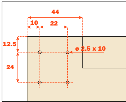
Lavorazione per il fissaggio del sistema sul fianco del mobile
