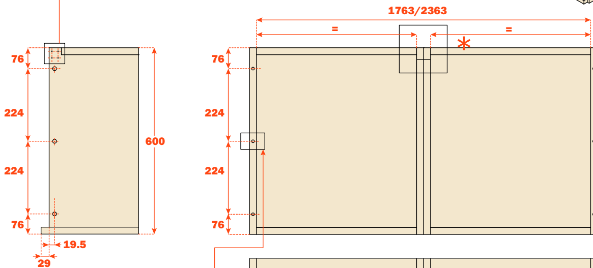
Lavorazione per il fissaggio del sistema sul fianco del mobile
