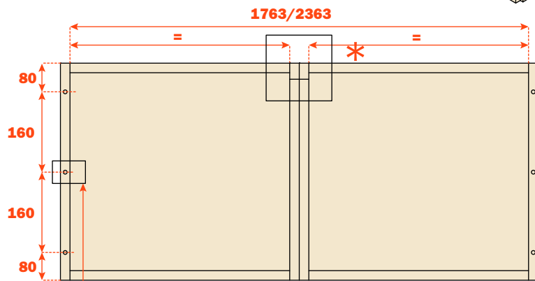
Lavorazione per il fissaggio del sistema sul fianco del mobile
