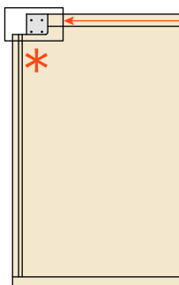
Lavorazione per il fissaggio della guida sul fianco da 19/20 mm
