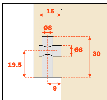
Lavorazione per il fissaggio della guida sul fianco da 18 mm
