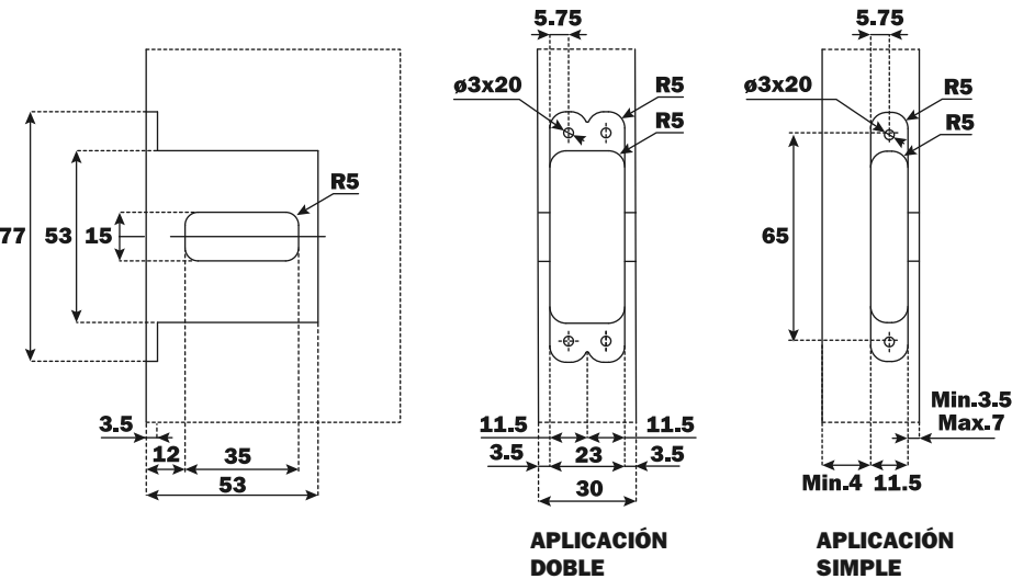
Solape D1 con aplicación simple
