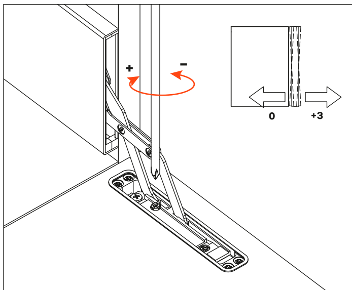
Ajuste frontal
