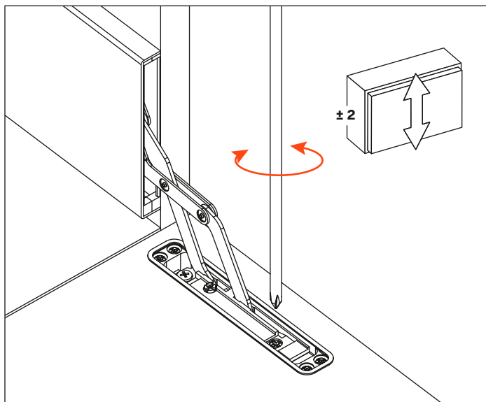
Ajuste frontal
