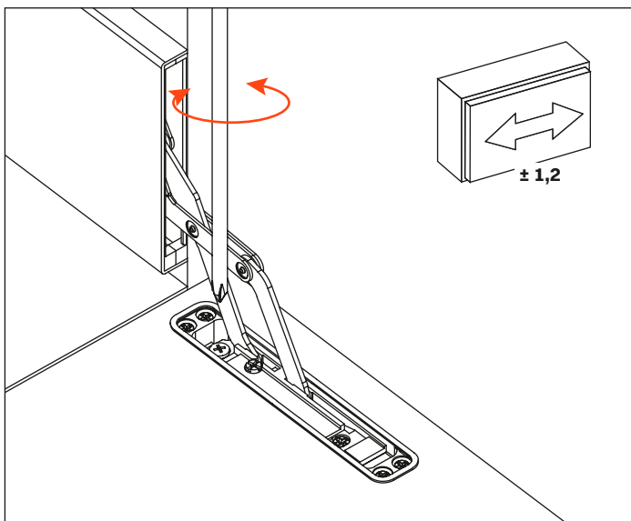
Ajuste lateral
