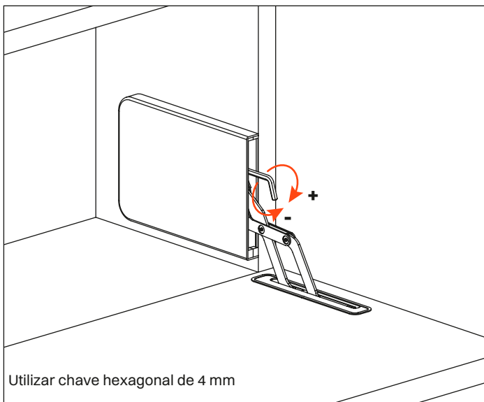
Ajuste lateral
