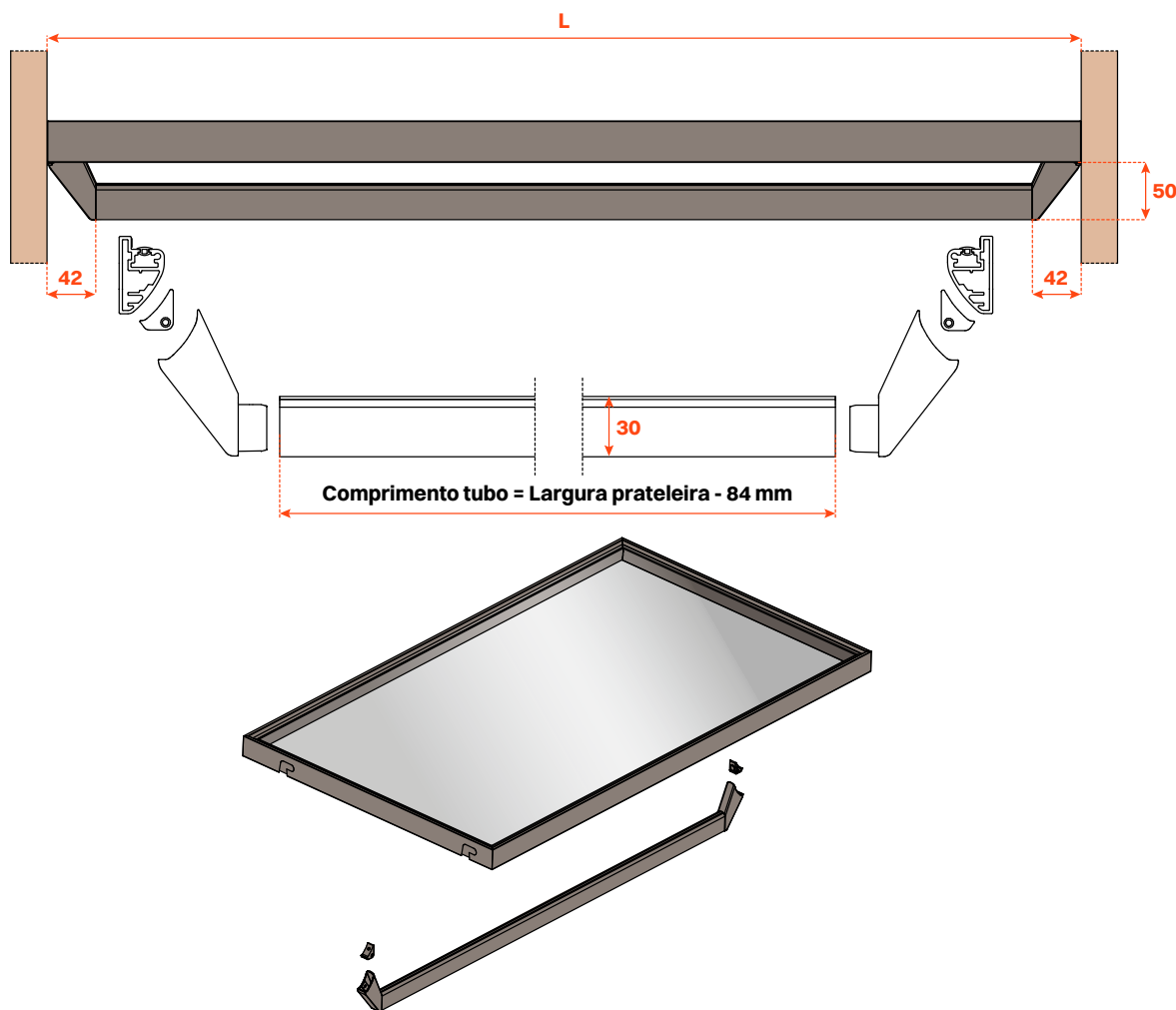
Parafusar os adaptadores na prateleira
