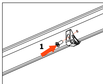
Parafusar os adaptadores na prateleira
