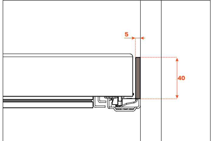
4. Mesures d'encombrement
