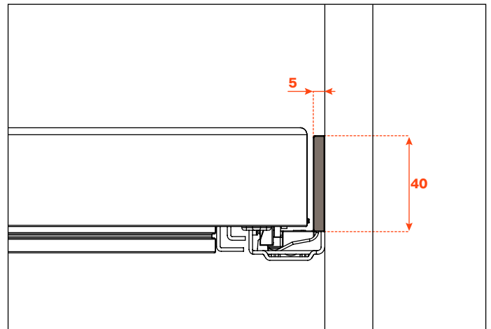
4. Misure d'ingombro
