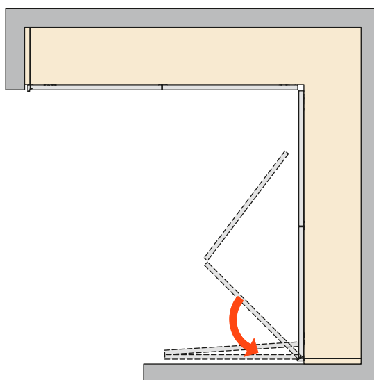
DOPPELSCHRANK
