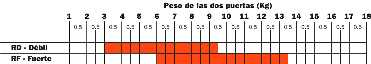
Altura total de las dos puertas da 570 a 630 mm
