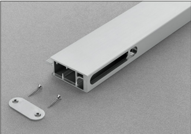
Perfil de soporte para bisagras - espesor 16 mm
