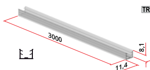
6716 Glasdichtung für 5-6 mm Glas
