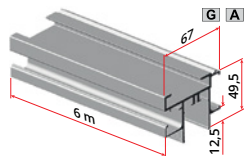
2421/19 Aluminiumprofil zur Befestigung der Schiene 2201 an der abgehängten Decke
