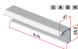
4204/41 Aluminiumprofil zur Wandbefestigung
