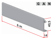
4240 Aluminium-Abdeckung
