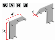
4211 Paar Nylon-Endkappen
