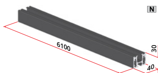
6710/N Horizontales Aluminiumprofil
